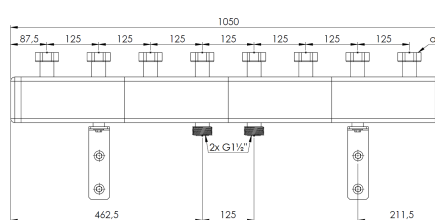
(a) - 8x nakrętka G1½"
